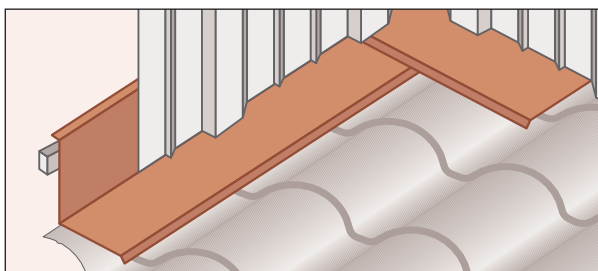
9. Vierendeaguas liso
