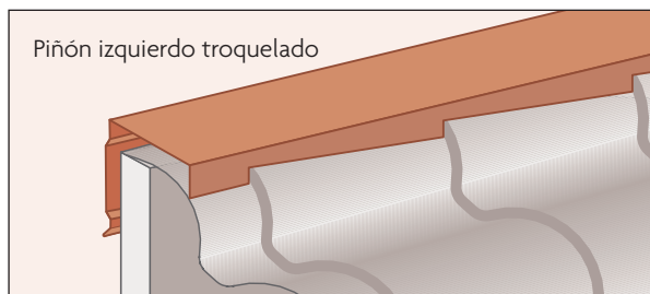
8. Piñón troquelado
