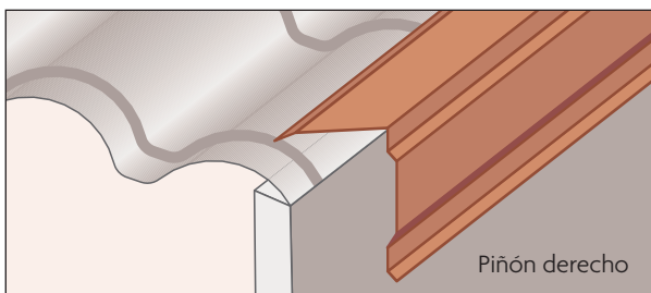
7. Piñón liso
