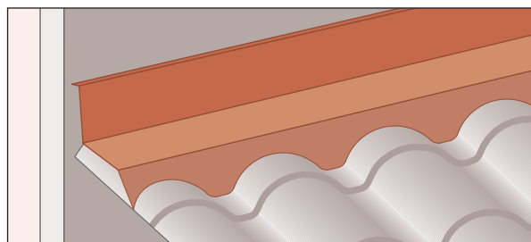
10. Vierendeaguas superior troquelado
