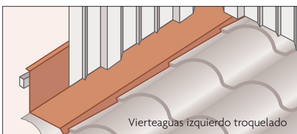
11. Vierendeaguas lateral troquelado
