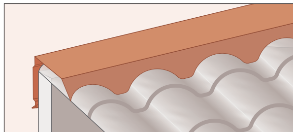
4. Cumbreira diente de sierra troquelada
