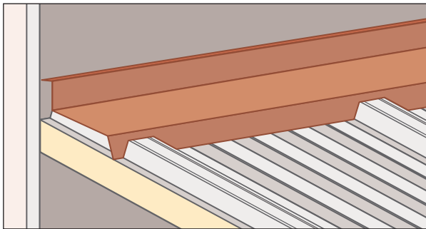
23. Vienteaguas troquelado superior panel
