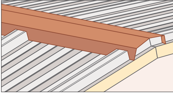
21. Cumbre troquelada panel
