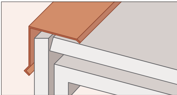
3. Cumbrera diente de sierra
