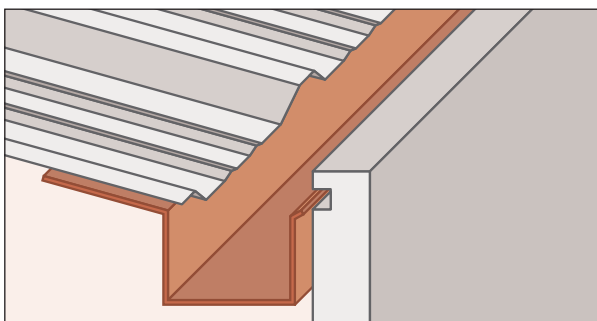
7. Canalón normal
