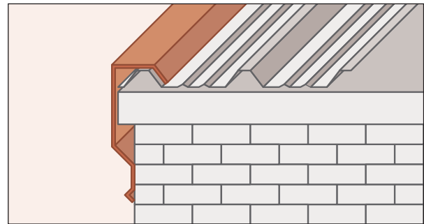
6. Cornisa
