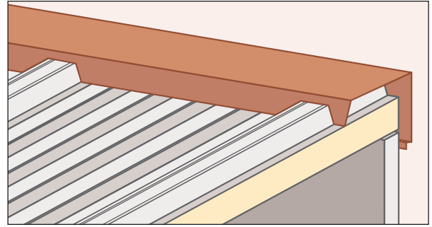
22. Cumbre troquelada diente de sierra panel
