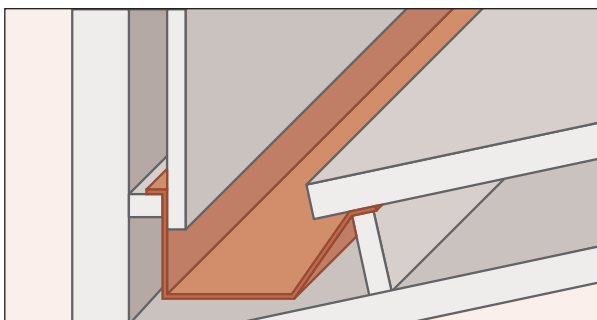
9. Canalón diente de sierra
