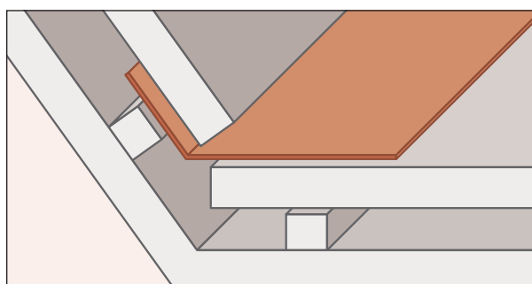
15. Lima frontal
