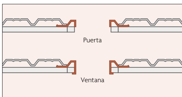
19. Jambas
