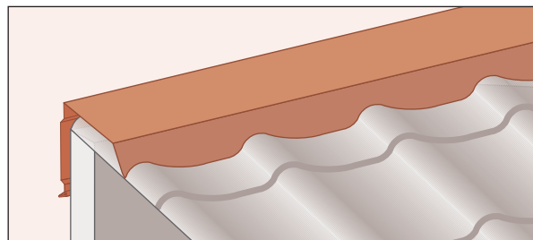
4. Cumbrera diente de sierra troquelada
