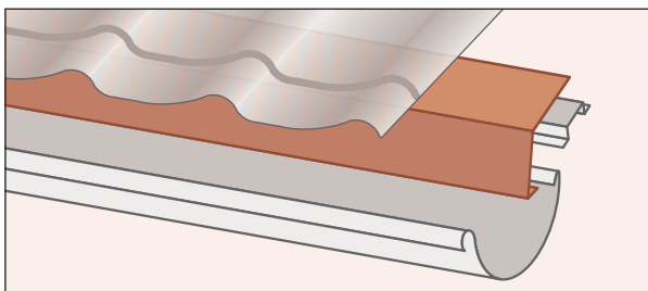
5. Alero
