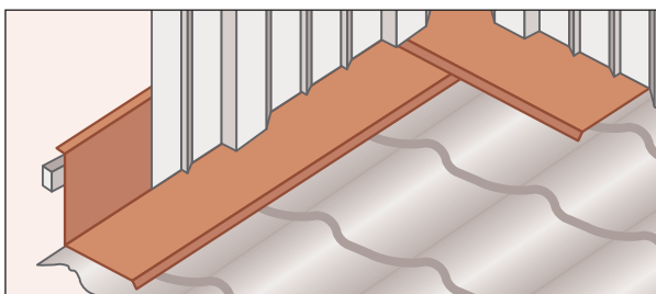
9. Vierendeaguas liso
